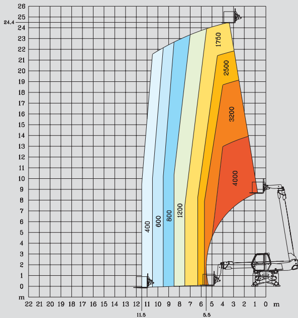
360° ABGESTÜTZT MIT JIB P600
