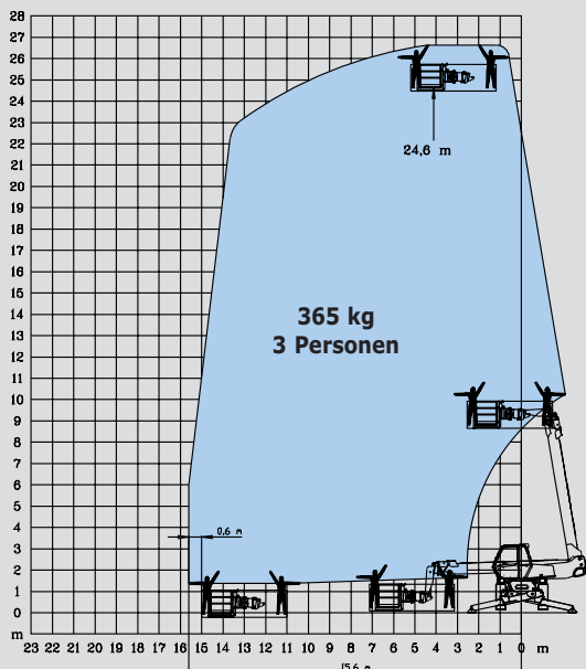
360° ABGESTÜTZT MIT ARBEITSBÜHNE VERSTELLBAR 2.25/4 m
