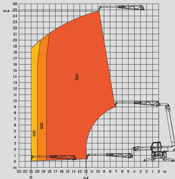
360° ABGESTÜTZT MIT TELESKOPIERBARER KRANARM
