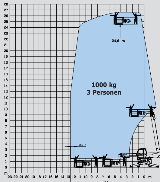
360° ABGESTÜTZT MIT ARBEITSBÜHNE VERSTELLBAR 1000 KG 2.25/4 m
