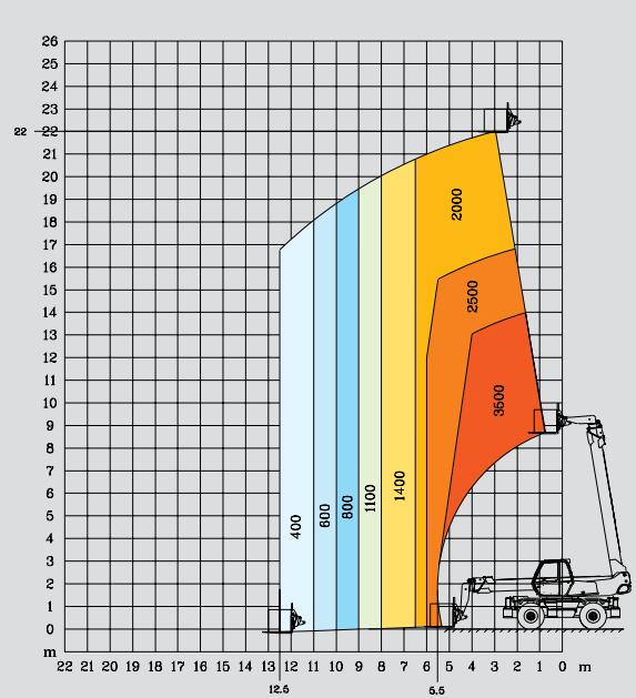
360° ABGESTÜTZT MIT SEILWINDE 5T
