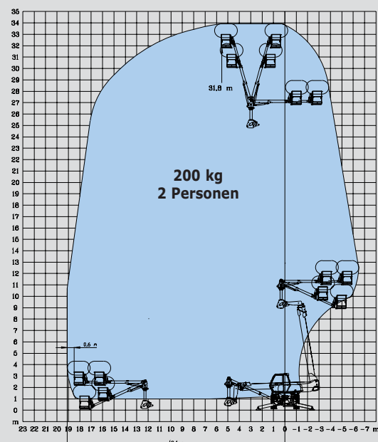
360° ABGESTÜTZT MIT TELESKOPIERBARER KRANARM
